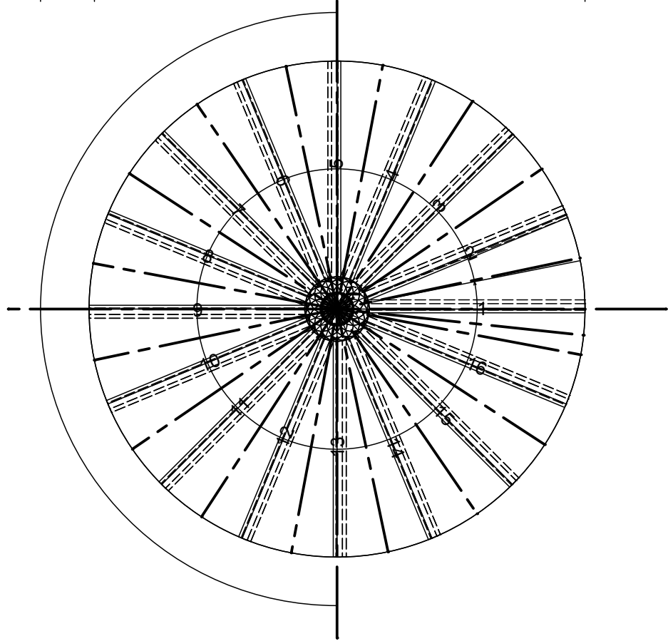
Escalier hélicoïdal à noyau décentré supportant une voûte dite "en palmier"
