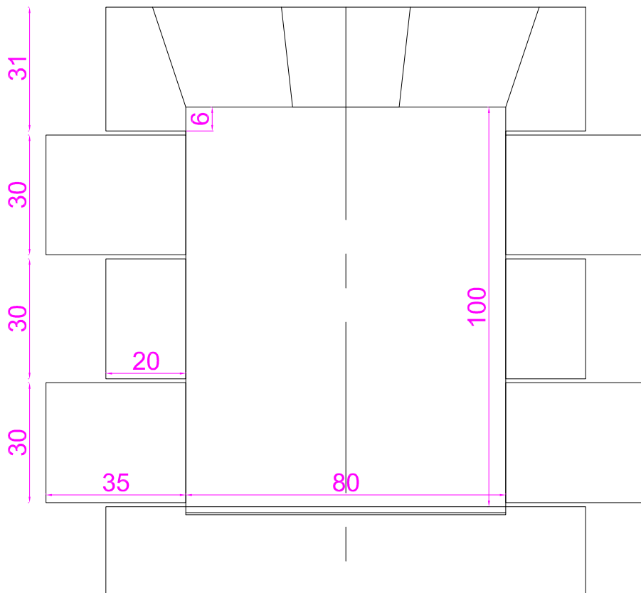
Elévation
