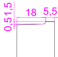
Coupe de l'appui
